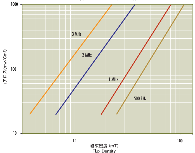
L材のコアロス (100 ^{\circ} C時)
